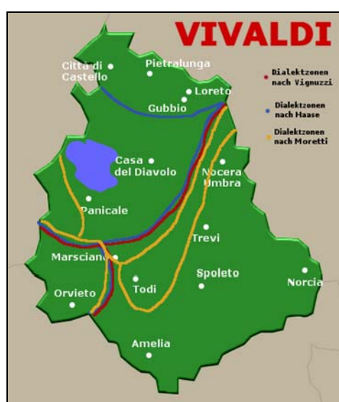
Abbildung 3: Dialektzonen in Umbrien
